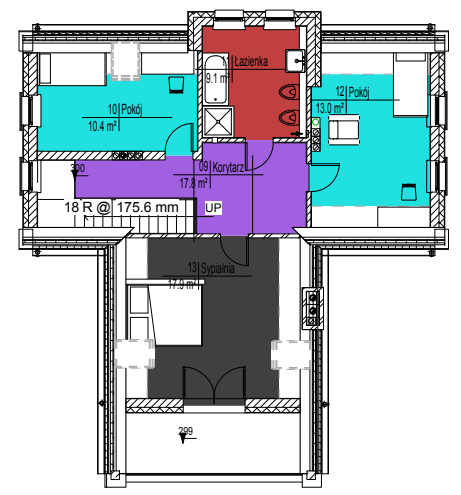
2 03 PODDASZE - pomieszczenia 1 : 100
