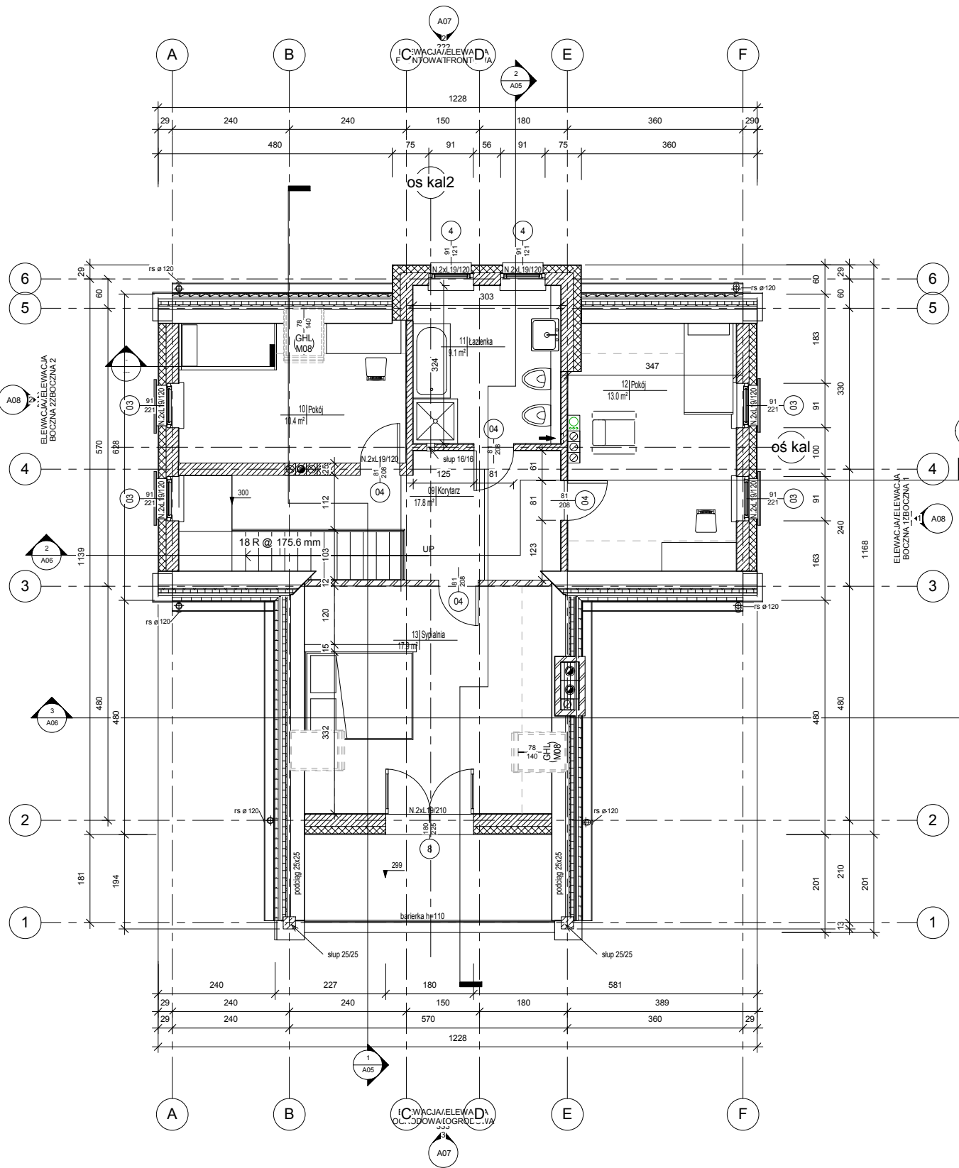
1 03 PODDASZE 1 : 50
