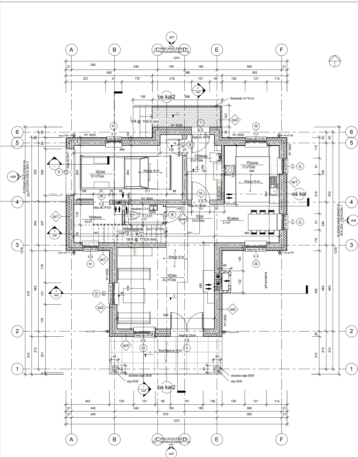
1 02 PARTER 1 : 50
