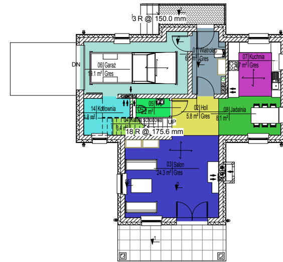
2 02 PARTER - pomieszczenia 1 : 100
