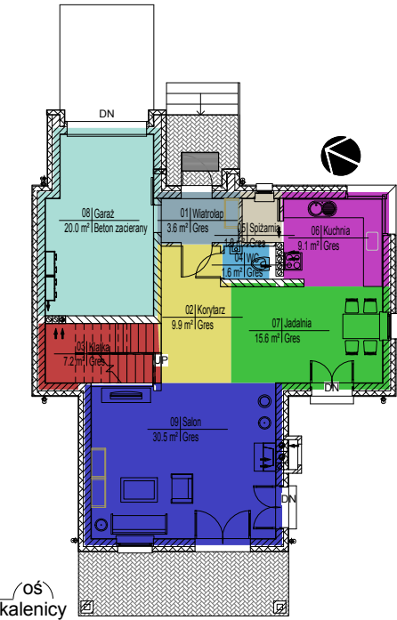
2 02 PARTER - pomieszczenia 1 : 100
